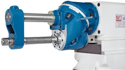
Horizontalfräseinrichtung (serienmäßig)
